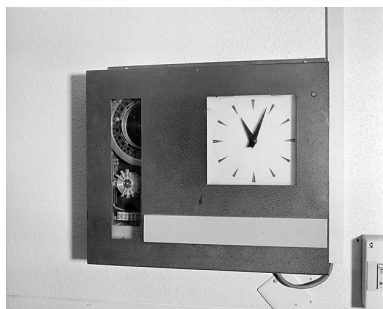
Horloge mère. Phot. Jérôme Mongreville IVR43_20023900150X
