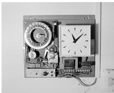
Horloge mère : modules sonnerie et garde-temps. Phot. Jérôme Mongreville IVR43_20023900149X
