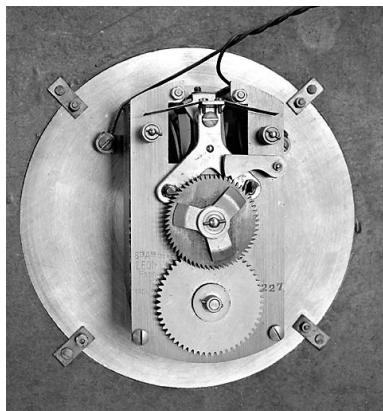
Horloge secondaire : système moteur.
