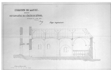
Commune de Lajoux. Restauration de l'église de Mijoux [coupe longitudinale de l'église]. Phot. Jérôme Mongreville, Phot. Auguste Comoy IVR43_19963901756X
