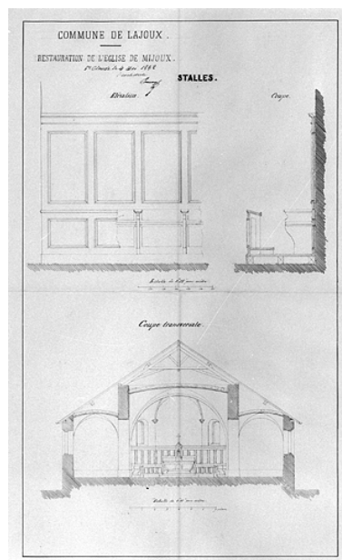
Commune de Lajoux. Restauration de l'église de Mijoux [élévation et coupe des stalles et coupe transversale de l'église].
