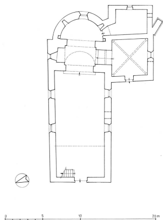
Plan. Dess. Alain Morelière IVR26_20122100524A3YY
