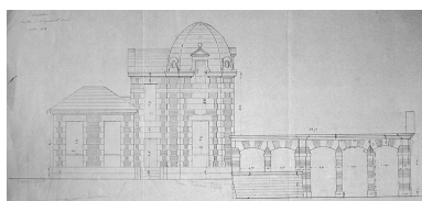
Pavillon de l'équatorial coudé [élévation latérale ouest : variante], 1883-1884. Phot. Yves Sancey IVR43_20042500207X
