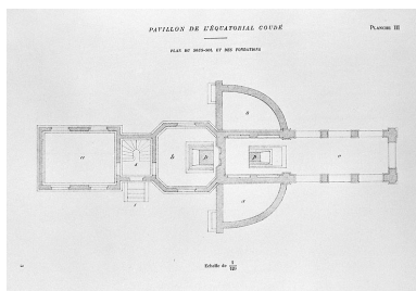
Pavillon de l'équatorial coudé. Plan du sous-sol et des fondations, 1892. Phot. Jérôme Mongreville, Autr. Auguste Hérique IVR43_20032500641X
