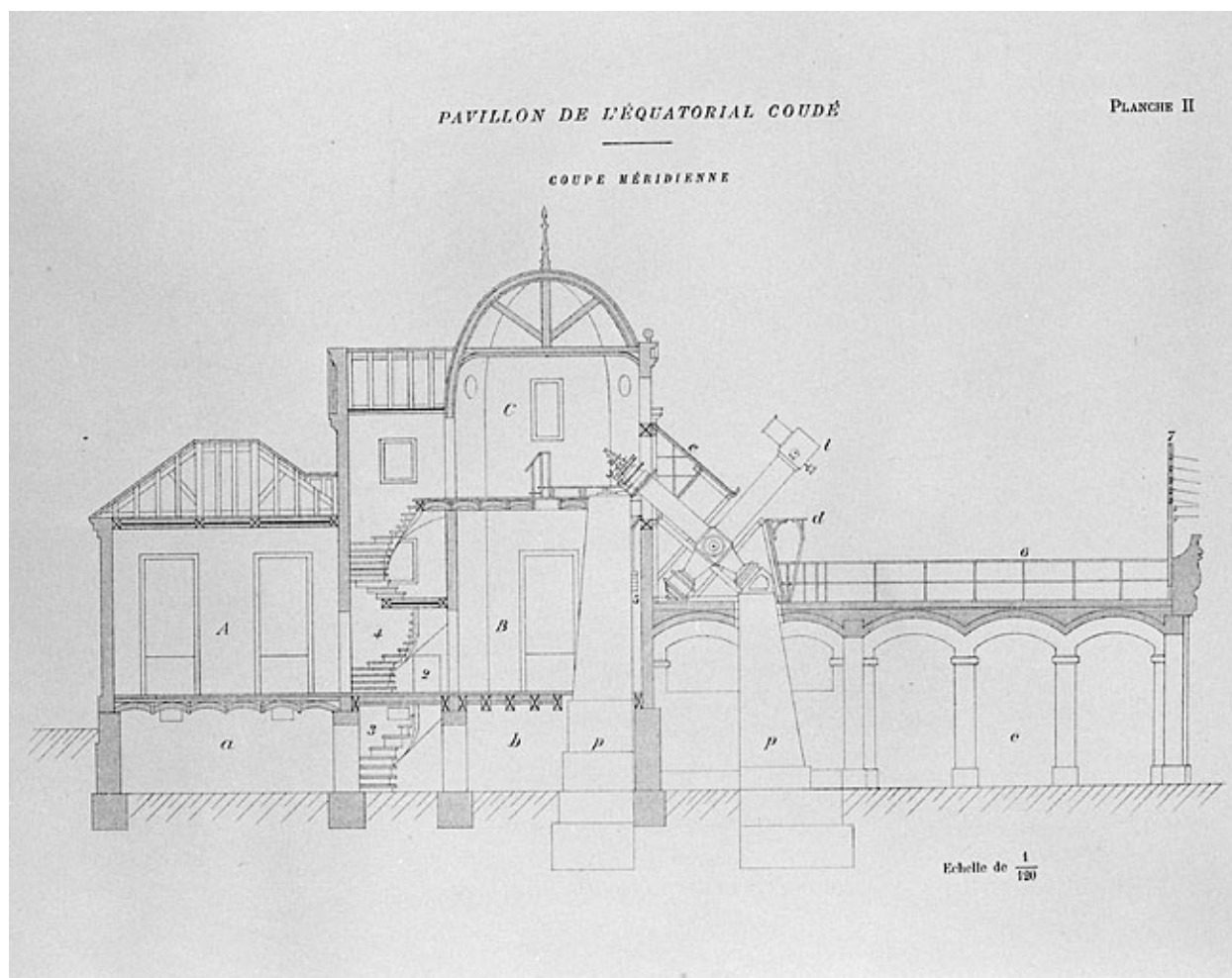
Pavillon de l'équatorial coudé. Coupe méridienne, 1892.
