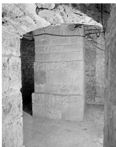
Sous-sol de la tour de l'équatorial coudé : vue d'ensemble du pilier de la lunette. Phot. Jérôme Mongreville IVR43_20022501147X
