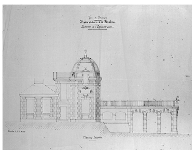
Ville de Besançon. Observatoire à la Bouloie. Bâtiment de l'équatorial coudé. Elévation latérale [variante de l'élévation ouest], 1883-1884. Phot. Jérôme Mongreville IVR43_20032500565V
