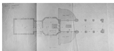
Pavillon de l'équatorial coudé. Rez-de-chaussée [plan], 1883-1884.
