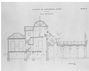
Pavillon de l'équatorial coudé. Coupe méridienne, 1892. Phot. Jérôme Mongreville, Autr. Auguste Hérique IVR43_20032500642X
