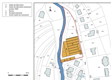
Plan-masse et de situation. Dess. Mathias Papigny IVR43_20132502628NUDA
