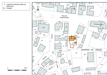
Plan-masse et de situation. Extrait du plan cadastral, 2015, section AE. Dess. Mathias Papigny IVR43_20152500705NUDA
