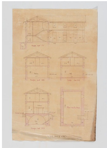
Projet pour une auberge ou un hôtel de voyageurs, coupes transversales et élévations sur la cour.
