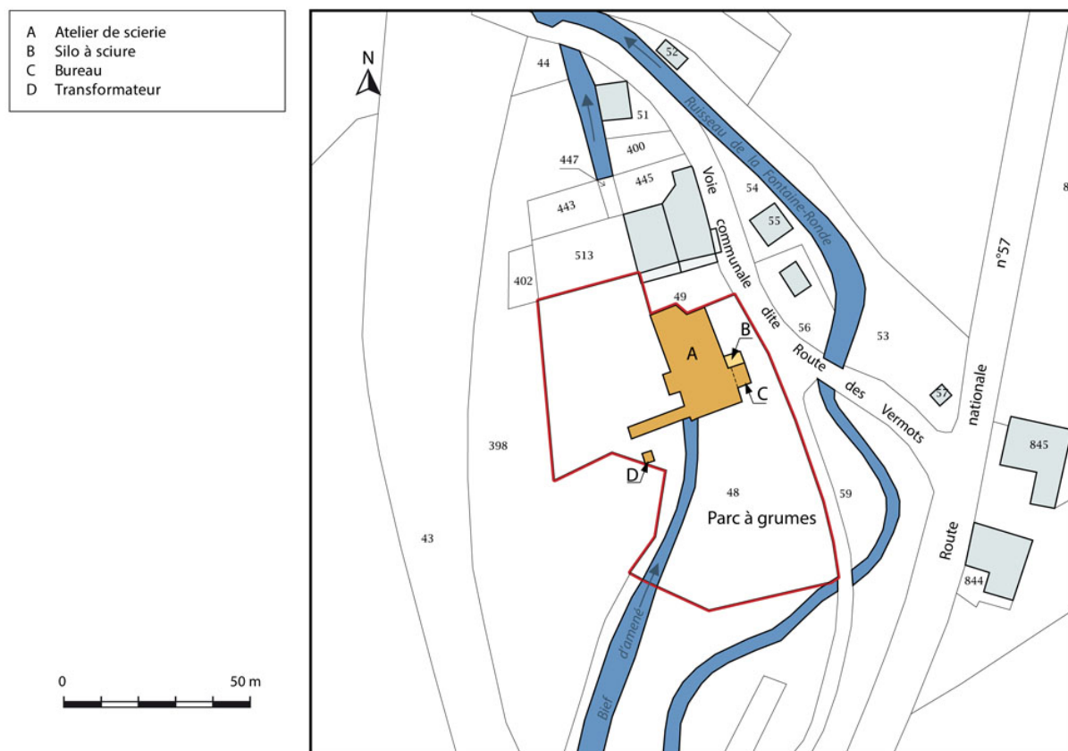
Plan-masse et de situation. Extrait du plan cadastral, 2015, section D.
