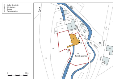
Plan-masse et de situation. Extrait du plan cadastral, 2015, section D. Dess. Mathias Papigny IVR43_20162500936NUDA
