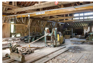
Intérieur de l'atelier de sciage. Phot. Jérôme Mongreville IVR43_20162500411NUC4A
