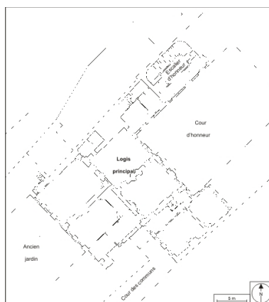
Plan de l'étage entre cour et jardin. Dessin original non numérique sur transparent synthétique. Dess. André Céréza, Autr. Muriel Sarfaty, Autr. Françoise Doutreuve IVR43_20092500836NUDA
