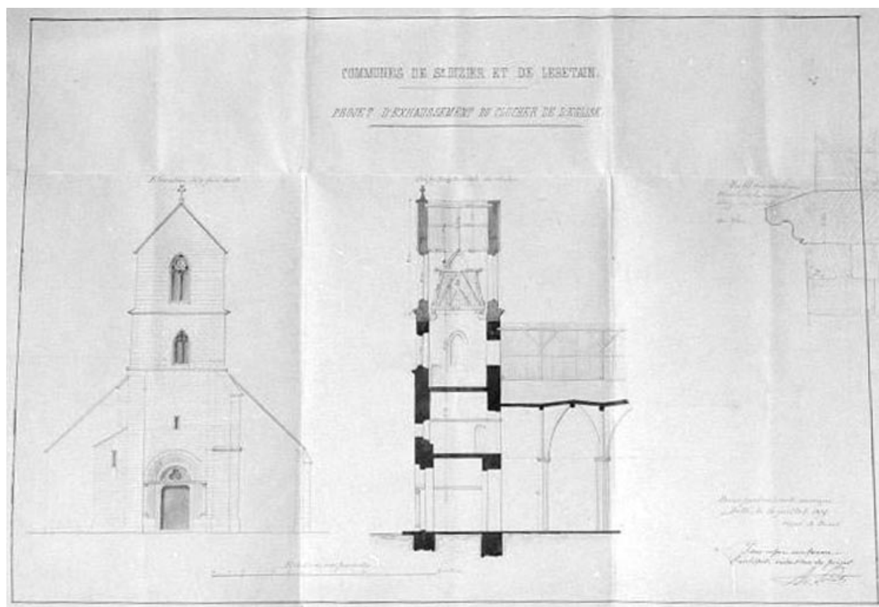
Projet d'exhaussement du clocher de l'église. Dessin par A. Poisat, 1875.
