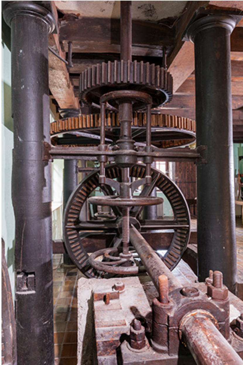
Arbre principal et système de transmission du beffroi est.
