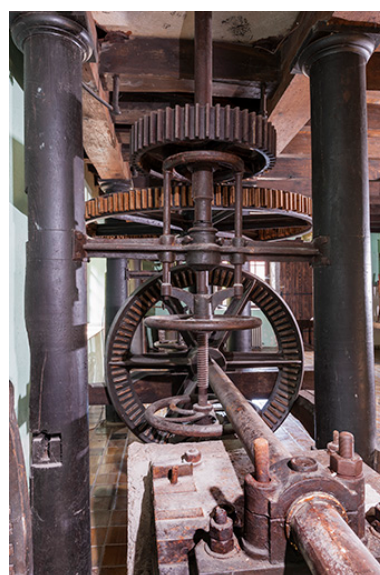
Arbre principal et système de transmission du beffroi est. Phot. Jérôme Mongreville IVR43_20152501748NUC4A
