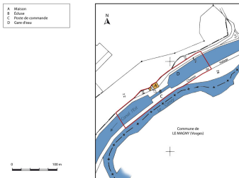
Plan masse et de situation. Dess. Mathias Papigny IVR43_20167000163NUDA
