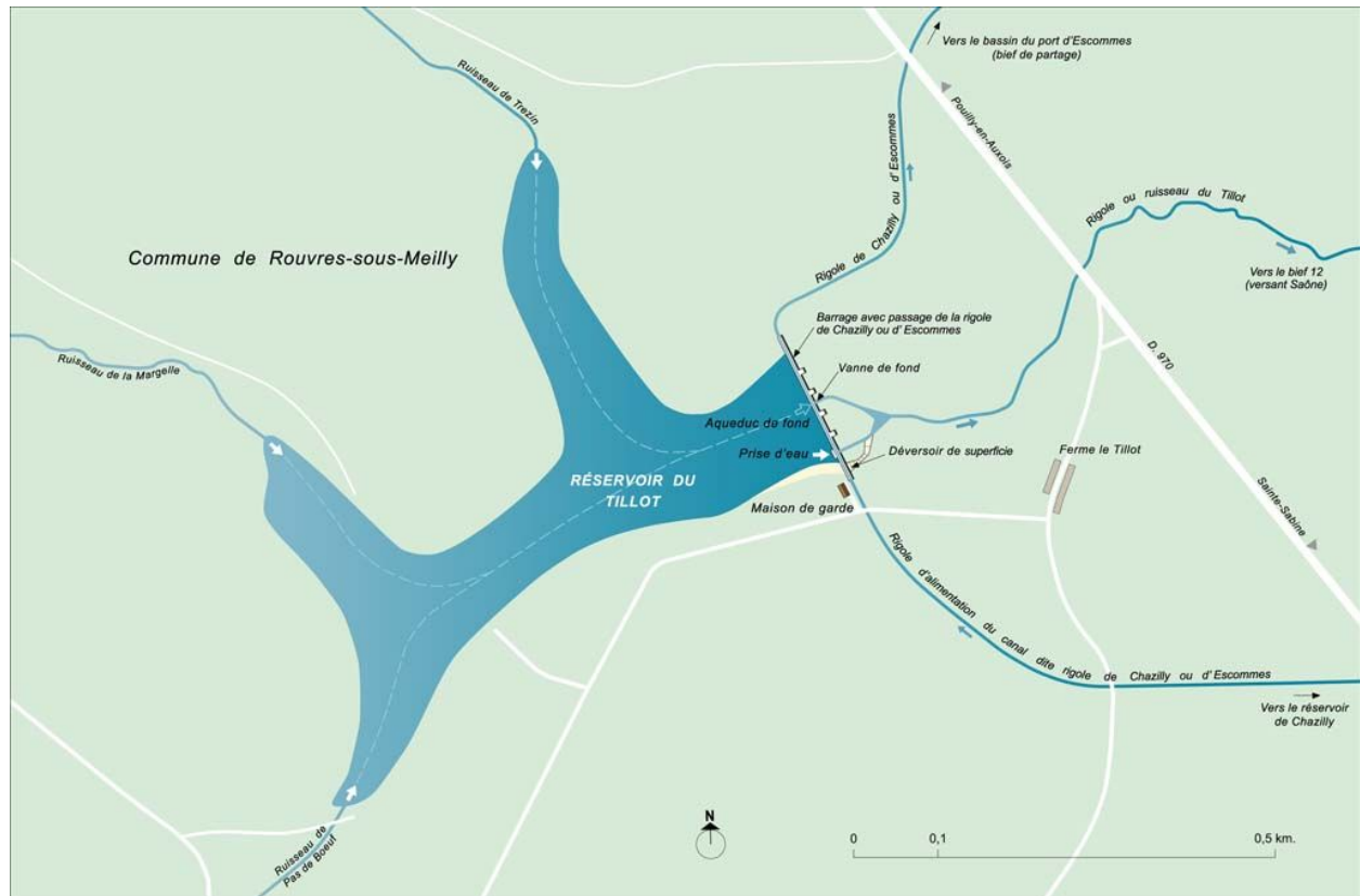
Plan du réservoir du Tillot.
