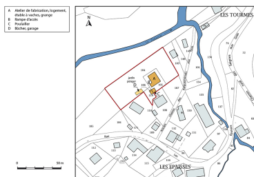
Plan-masse et de situation. Extrait du plan cadastral, 2017, section AB, 1/1 000. Dess. Mathias Papigny IVR43_20172501277NUDA
