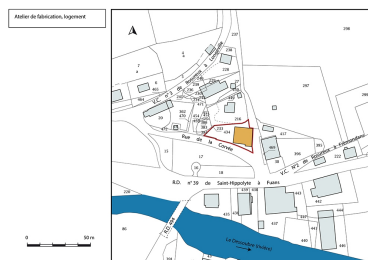
Plan-masse et de situation. Extrait du plan cadastral, 2018, section B. Dess. Bertrand Turina IVR43_20202500290NUDA
