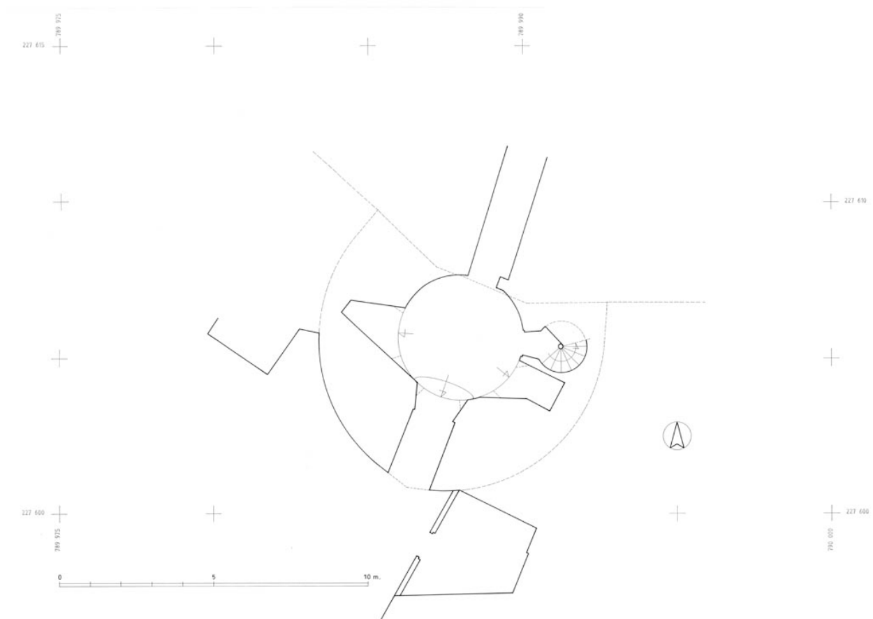
Tour des Cordeliers. Plan du premier niveau.
