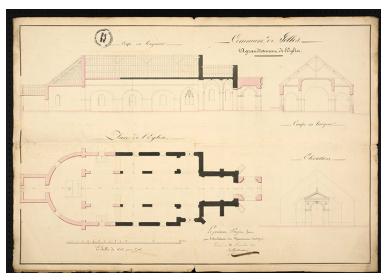
Plan de l'agrandissement de l'église (1827).
