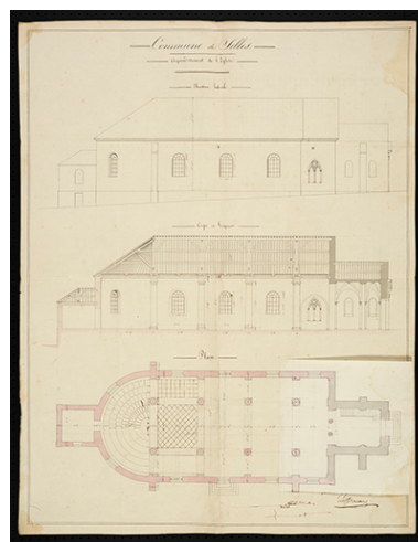
Plan de l'agrandissement de l'église (1827).
