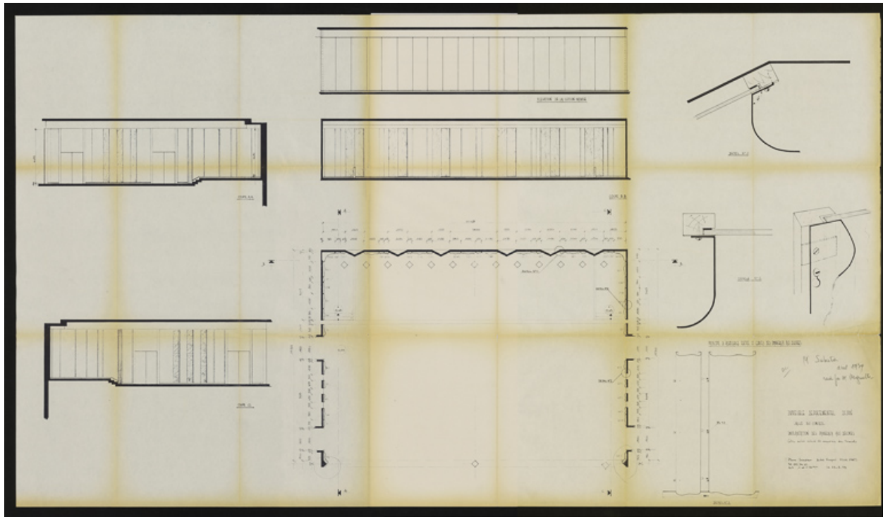
Salle des assemblées: plan de répartition des panneaux en aluminium, élévations des murs et détails de fixation, 23 mars 1979. Boyer, Michel (architecte d'intérieur) (Archives départementales de la Côte-d'Or, Dijon, 32 J 82)
