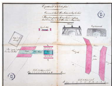
Plan d'un pontceau et d'un abreuvoir à construire dans la
