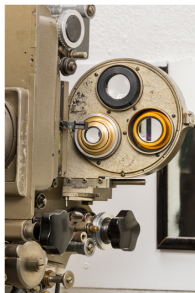
Tourelle à trois objectifs. Phot. Pierre-Marie Barbe-Richaud IVR26_20245800398NUC4A
