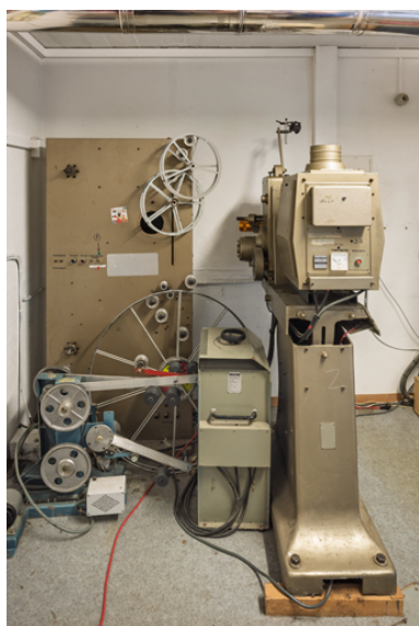
Vue d'ensemble de dos, avec le redresseur IREM et le dérouleur de film. Phot. Pierre-Marie Barbe-Richaud IVR26_20245800396NUC4A
