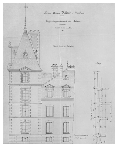
Projet d'agrandissement du château. Monsieur Armand Viellard à Morvillars. Façade latérale du sud-est. Phot. Jérôme Mongreville, Phot. Anthime Fleury de la Hussinière IVR43_20019000049V
