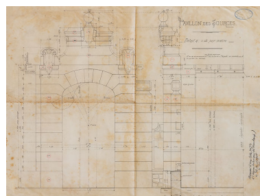
Élévation et coupe de la façade en pierre de taille de la partie sud (1905). Phot. Pierre-Marie Barbe- Richaud, Autr. Charles Arnaud IVR26_20205800200NUC4A
