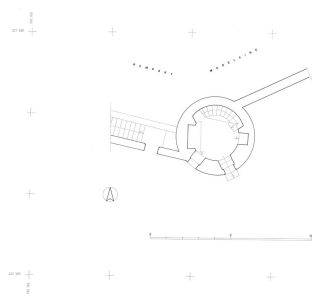
Tour des Billes. Plan du niveau supérieur. Dess. Alain Morelière IVR26_20122100090A3YY
