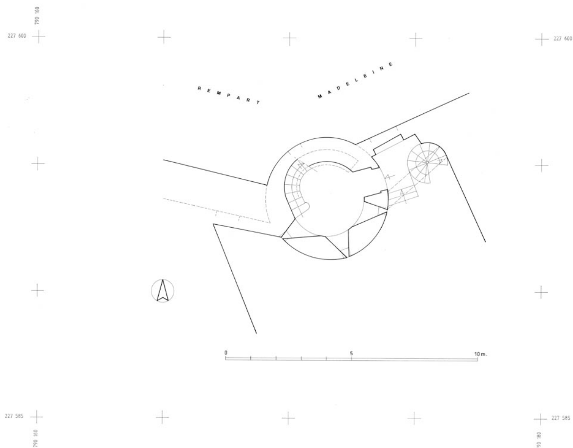
Tour des Billes. Plan du niveau inférieur.
