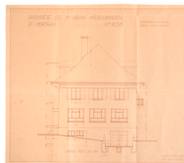
Propriété de Mr Henri Michel-Amadry, à Morteau. Façade ouest, février 1930. Phot. Sonia Dourlot IVR43_20182500489NUC4A
