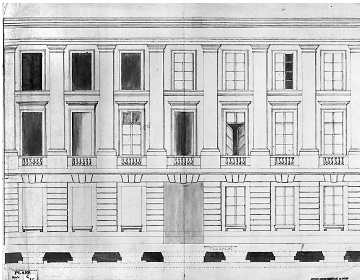
Elévation de la façade sur rue.
