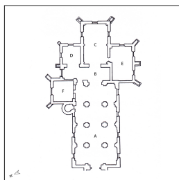
Plan avec la localisation des chapelles. Dess. Aline Thomas IVR26_20237100085NUDA
