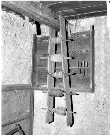
Rateliers. Le ratelier du second plan accueille les outils du tourneur, celui du premier plan (portant des axes) semble ne pas avoir de lien avec le tour. Phot. Jérôme Mongreville IVR43_19943901211X
