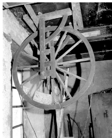
Roue motrice au plafond. Phot. Jérôme Mongreville IVR43_19943901213X
