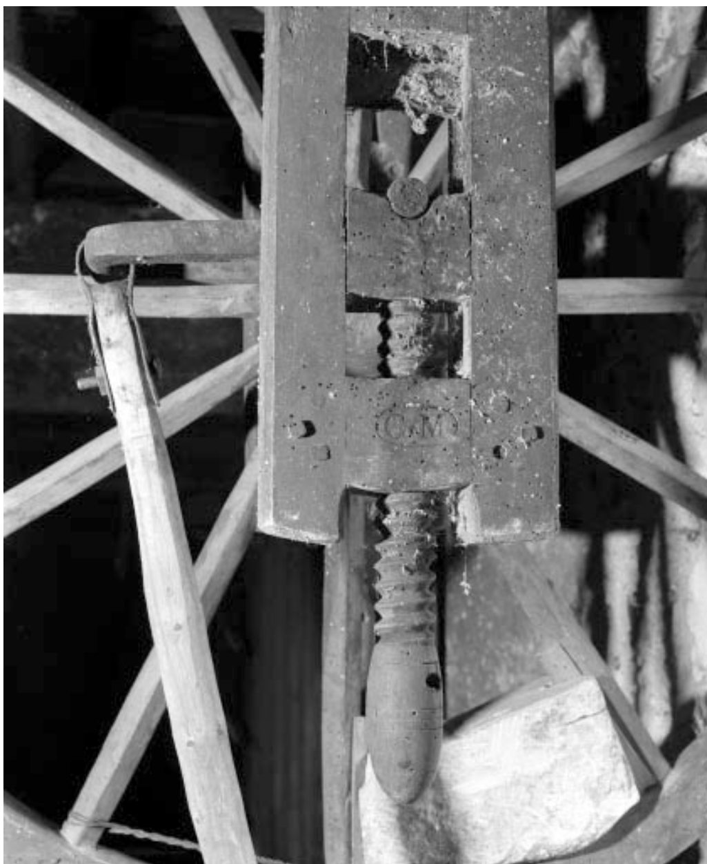
Vis de réglage en hauteur de l'axe de la roue et inscription.
