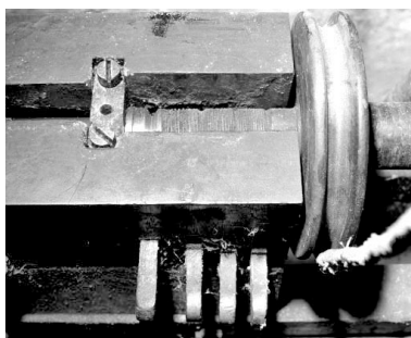
Détail du filetage de l'arbre du tour et des clés de sélection. Phot. Jérôme Mongreville IVR43_19943901216X
