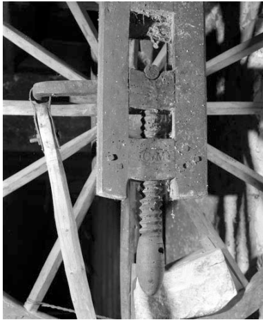
Vis de réglage en hauteur de l'axe de la roue et inscription. Phot. Jérôme Mongreville IVR43_19943901214X
