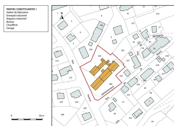
Plan-masse et de situation. Extrait du plan cadastral, 2013, section AE. Dess. Mathias Papigny IVR43_20142501519NUDA
