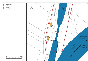
Plan masse et de situation. Dess. Bertrand Turina IVR43_20207000775NUDA
