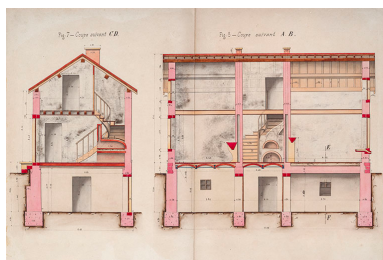
Bief de Chantes. Construction d'une dérivation éclusée, d'un barrage mobile et d'un chemin de halage - Maisons éclusières, plans, coupes, élévation et détails (1878) : vues en coupe. Phot. Jérôme Mongreville, Autr. Gustave Bouvaist IVR43_20207000087NUC4A
