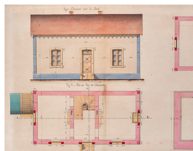
Bief de Chantes. Construction d'une dérivation éclusée, d'un barrage mobile et d'un chemin de halage - Maisons éclusières, plans, coupes, élévation et détails (1878) : élévation sur canal. Phot. Jérôme Mongreville, Autr. Gustave Bouvaist
