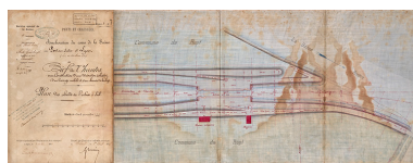
Bief de Chantes. Construction d'une dérivation éclusée, d'un barrage mobile et d'un chemin de halage - Plan des abords de l'écluse à sas (1878). Phot. Jérôme Mongreville, Autr. Gustave Bouvaist IVR43_20207000084NUC4A
