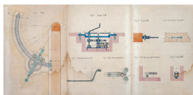
Bief de Chantes. Construction d'une dérivation éclusée, d'un barrage mobile et d'un chemin de halage - Ecluse à sas, détails de l'appareil de manoeuvre des portes (1878). Phot. Jérôme Mongreville, Autr. Gustave Bouvaist IVR43_20207000085NUC4A
