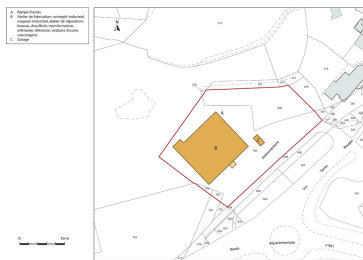
Plan-masse et de situation. Dess. Mathias Papigny IVR43_20162501486NUDA
