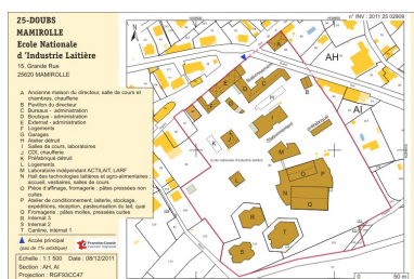
Plan-masse et de situation. Extrait du plan cadastral numérisé, sections AH et AI, échelle 1:1500. Dess. André Céréza IVR43_20112502909NUDA
