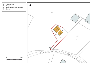
Plan-masse et de situation. Extrait du plan cadastral, 2016, section G, 1/2 500 agrandi à 1/1 000.
