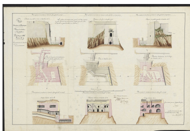
Place de Salins (fort Belin). Projets pour 1826. Reconstruction du cavalier. Autr. Perreau IVR43_20223901203NUC4A
