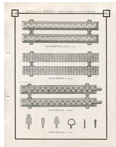
Planchettes et chevilles. Dessin., s.n., s.d. [début du 20e siècle] Phot. Raphaël Favereaux, Autr. IVR43_20122501873NUC4A
