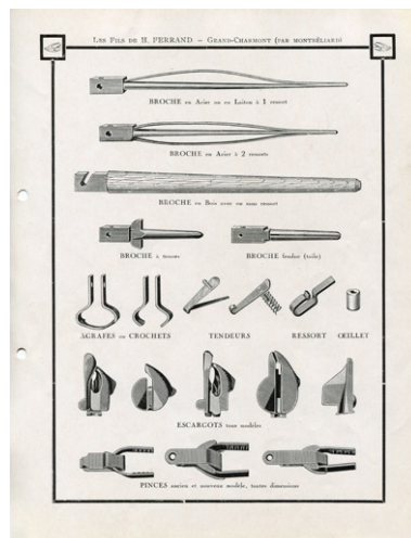
Broches, agrafes, tendeurs, ressorts, oeilletons, escargots, pinces. Dessin., s.n., s.d. [début du 20e siècle] Phot. Raphaël Favereaux, Autr. IVR43_20122501872NUC4A
