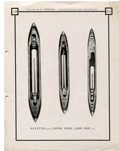
Navettes pour coton, toile, laine, soie, etc. Dessin., s.n., s.d. [début du 20e siècle] Phot. Raphaël Favereaux, Autr. IVR43_20122501870NUC4A
