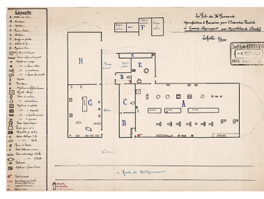
Plan de la manufacture d'accessoires pour l'industrie textile H. Ferrand, 1923.
