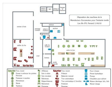
Disposition des machines de la Manufacture d'accessoires pour l'industrie textile Les fils d'H. Ferrand. D'après un croquis de 1923, conservé aux AD Doubs (M 1657). Dess. Mathias Papigny IVR43_20142500592NUDA
