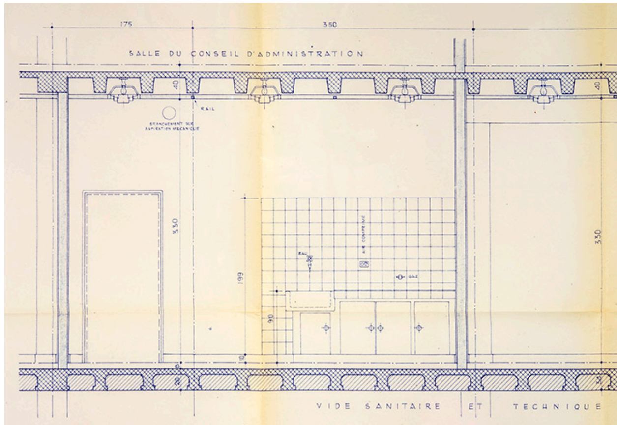
Cetehor Besançon. Construction du centre de l'industrie horlogère. 2008. Détails chambre noire et groupes standard des laboratoires. Rez-de-ch. inférieur [détail], 14 mars 1958.
