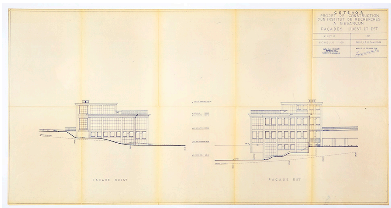
Projet de construction d'un institut de recherches à Besançon. 112. Façades ouest et est, 11 janvier 1958 (modifié le 25 mars 1958).
