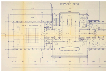
Projet de construction d'un institut de recherches à Besançon. 106. Plan du rez-de-chaussée supérieur [détail : hall et salles de conférence et du conseil d'administration], 11 janvier 1958. Phot. Sonia Dourlot, Autr. Denis Honegger IVR43_20192500021NUC4A
