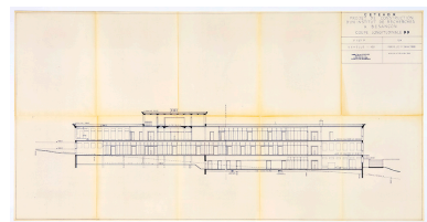
Projet de construction d'un institut de recherches à Besançon. 109. Coupe longitudinale D-D, 11 janvier 1958 (modifié le 25 mars 1958). Phot. Sonia Dourlot, Autr. Denis Honegger IVR43_20192500026NUC4A
