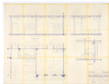
Cetehor Besançon. Construction du centre de l'industrie horlogère. 2008. Détails chambre noire et groupes standard des laboratoires. Rez-de-ch. inférieur, 14 mars 1958. Phot. Sonia Dourlot, Autr. Denis Honegger IVR43_20192500031NUC4A
