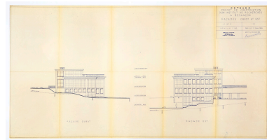
Projet de construction d'un institut de recherches à Besançon. 112. Façades ouest et est, 11 janvier 1958 (modifié le 25 mars 1958). Phot. Sonia Dourlot, Autr. Denis Honegger IVR43_20192500029NUC4A
