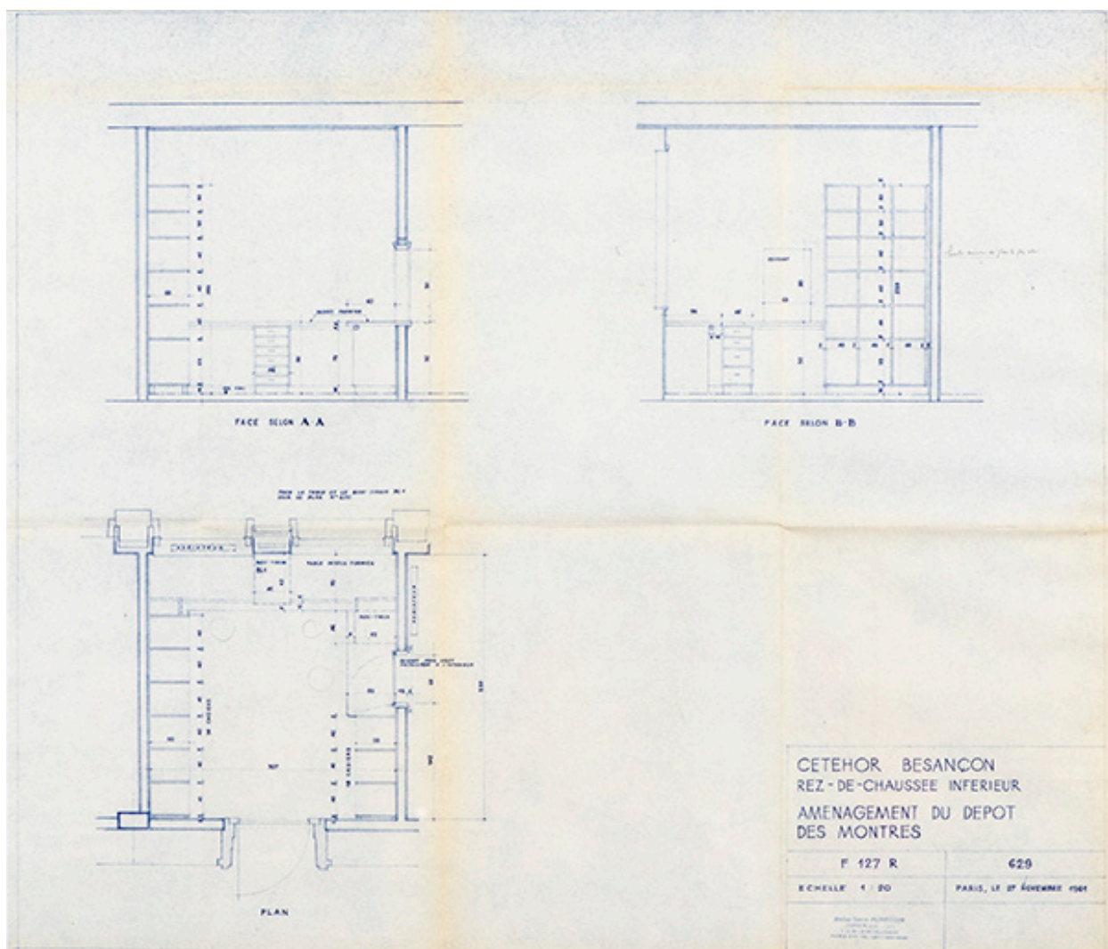
Cetehor Besançon. Rez-de-chaussée inférieur. 629. Aménagement du dépôt des montres, 27 novembre 1961.
