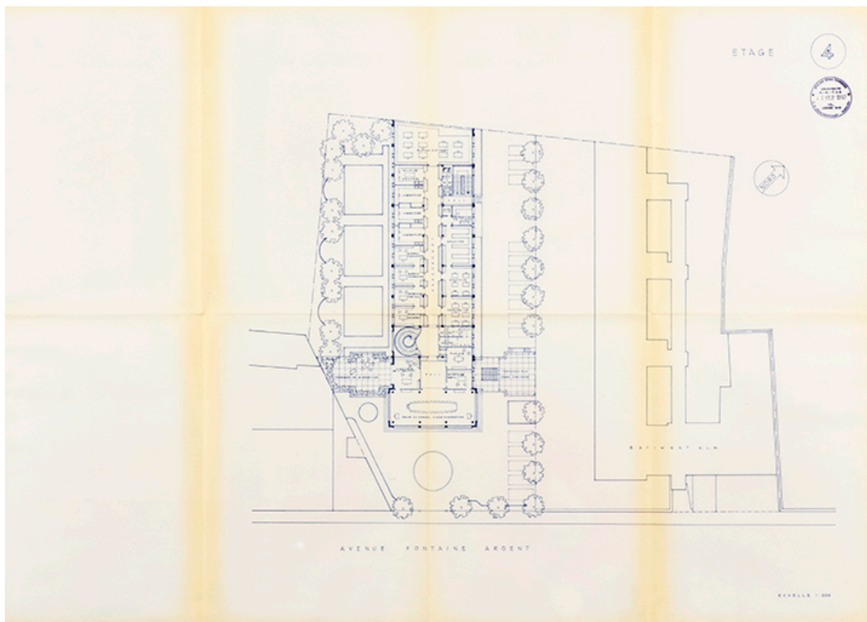
[Avant-projet Honegger avenue Fontaine-Argent]. 4. Etage, 16 septembre 1957.
