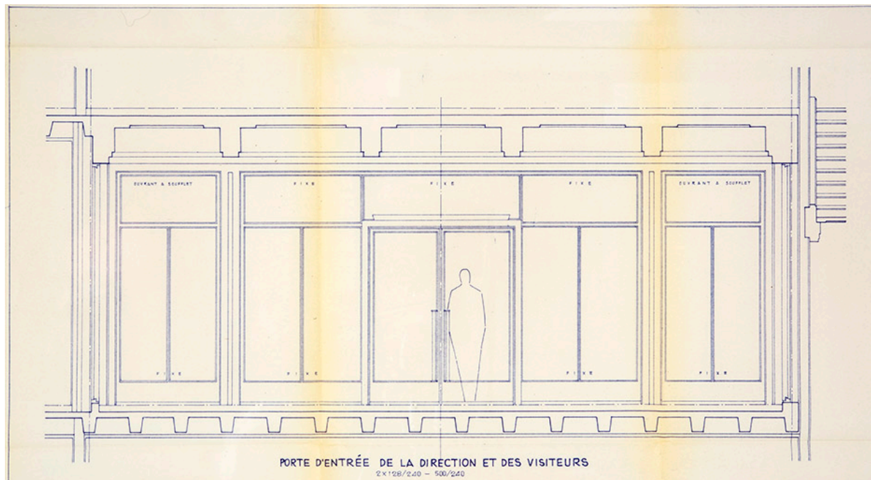
Cetehor Besançon. Construction du centre de l'industrie horlogère. 2016. Serrurie [sic] extérieure-intérieure [détail :] Porte d'entrée de la direction et des visiteurs, 12 mai 1958.
