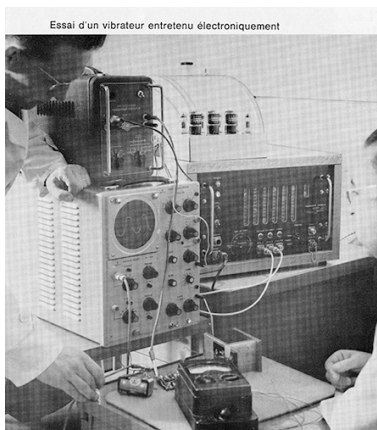
Essai d'un vibreur entretenu électroniquement, 1964.
