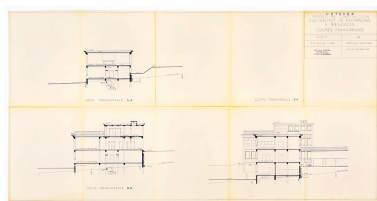
Projet de construction d'un institut de recherches à Besançon. 108. Coupes transversales, 11 janvier 1958 (modifié le 25 mars 1958). Phot. Sonia Dourlot, Autr. Denis Honegger IVR43_20192500024NUC4A
