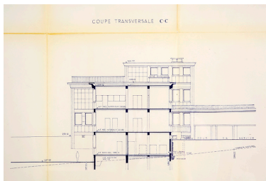
Projet de construction d'un institut de recherches à Besançon. 108. Coupes transversales [détail :] Coupe transversale C-C, 11 janvier 1958 (modifié le 25 mars 1958). Phot. Sonia Dourlot, Autr. Denis Honegger IVR43_20192500025NUC4A
