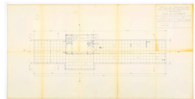
Projet de construction d'un institut de recherches à Besançon. 107. Plan de la terrasse, 11 janvier 1958. Phot. Sonia Dourlot, Autr. Denis Honegger IVR43_20192500023NUC4A
