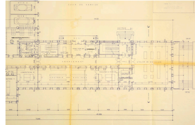
Projet de construction d'un institut de recherches à Besançon. 105. Plan du rez-de-chaussée inférieur [détail : contrôle des montres et atelier de mécanique], 11 janvier 1958. Phot. Sonia Dourlot, Autr. Denis Honegger IVR43_20192500019NUC4A
