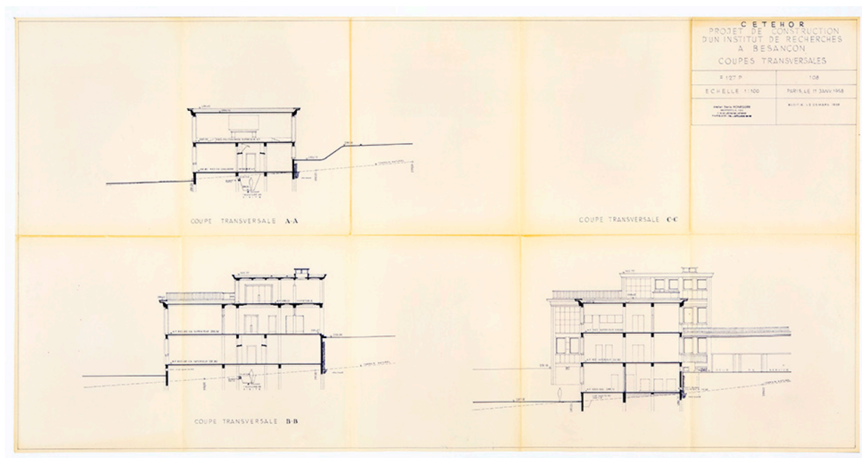
Projet de construction d'un institut de recherches à Besançon. 108. Coupes transversales, 11 janvier 1958 (modifié le 25 mars 1958).
