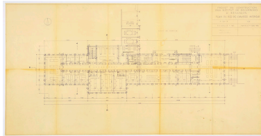
Projet de construction d'un institut de recherches à Besançon. 105. Plan du rez-de-chaussée inférieur, 11 janvier 1958. Phot. Sonia Dourlot, Autr. Denis Honegger IVR43_20192500020NUC4A
