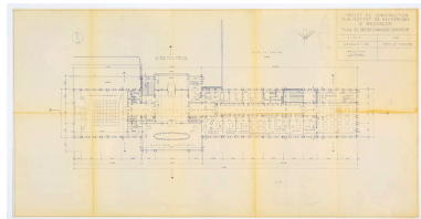
Projet de construction d'un institut de recherches à Besançon. 106. Plan du rez-de-chaussée supérieur, 11 janvier 1958. Phot. Sonia Dourlot, Autr. Denis Honegger IVR43_20192500022NUC4A
