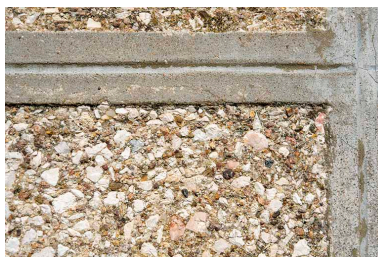
Détail de panneaux : aspect de surface et joints. Phot. Sonia Dourlot IVR43_20192500219NUC4A
