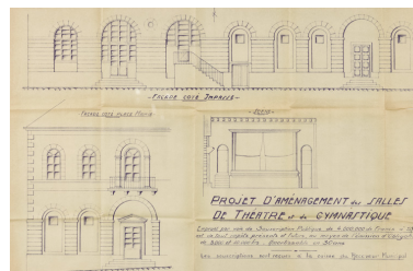
Projet d'aménagement des salles de théâtre et de gymnastique [coupe et élévations]. S.d. [1948]. Phot. Pierre-Marie Barbe- Richaud, Autr. Armand Inconnu IVR26_20245800371NUC4A
