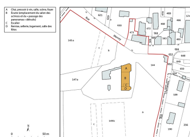
Plan-masse et de situation. Source : Direction générale des Finances Publiques - Cadastre ; mise à jour 2021, section D, 1/1 250 agrandi à 1/1 000. Dess. Aline Thomas IVR26_20222100292NUDA
