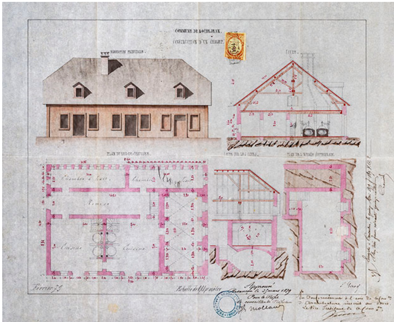
Construction d'un chalet [plans, coupes, élévation], 1879.
