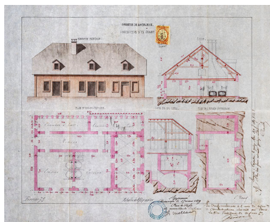
Construction d'un chalet [plans, coupes, élévation], 1879.
