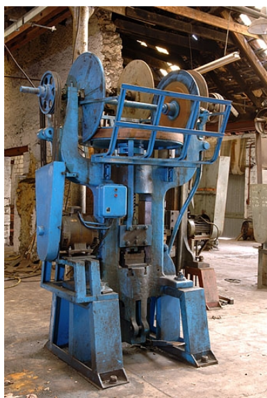
Vue de trois quarts d'une presse (D sur le plan de localisation). Phot. Jérôme Mongreville IVR43_20057000093NUCA
