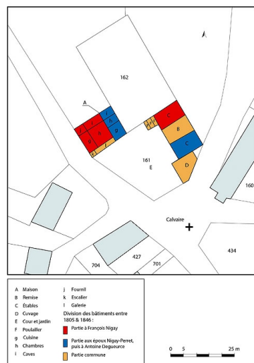
Plan de masse et de situation, présentant l'évolution des bâtiments. Extrait du plan cadastral, 2020, section B, échelle 1/2500 Dess. Pierre-Marie Barbe-Richaud IVR26_20207100131NUDA
