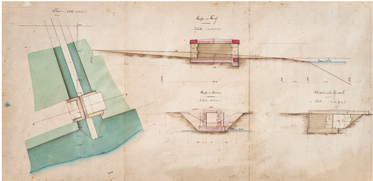
Projet de construction d'un aqueduc sous le chemin de halage (1877).
