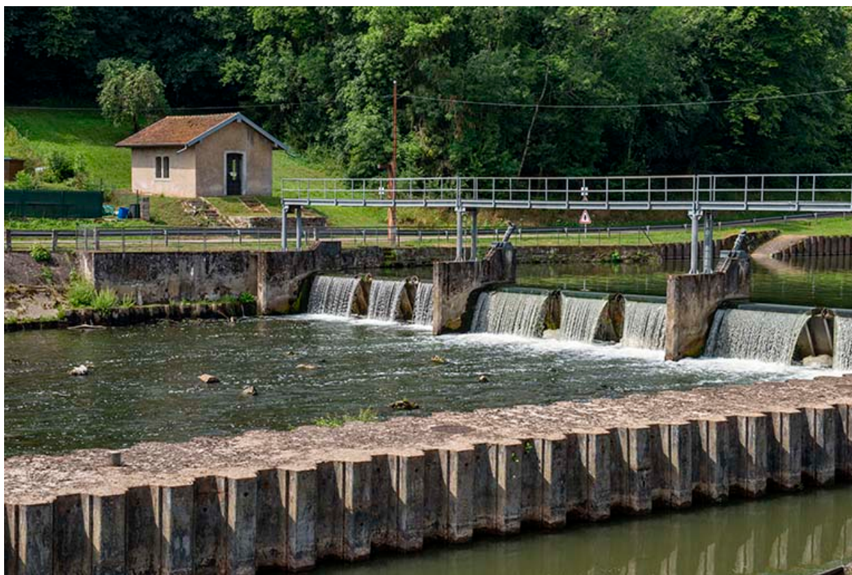
Le barrage mobile.
