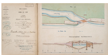
Passerelle de halage de 8m sur la Noue rouge (1877). Phot. Jérôme Mongreville, Autr. Charles Marie Albert Travelet IVR43_20207000171NUC4A
