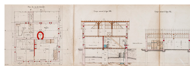
Dérivation de Conflandey : maison éclusière (1876). Phot. Jérôme Mongreville, Autr. Charles Marie Albert Travelet IVR43_20207000163NUC4A
