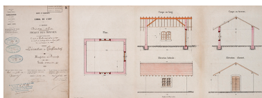
Magasin du barrage (1876). Phot. Jérôme Mongreville, Autr. Charles Marie Albert Travelet IVR43_20207000165NUC4A
