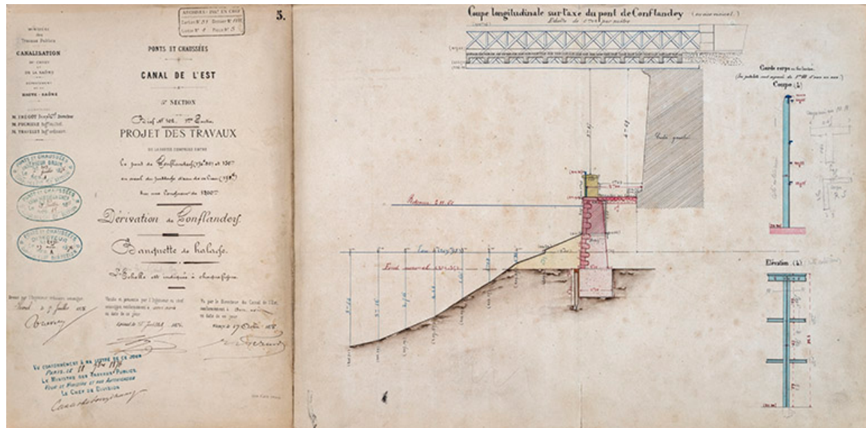
Dérivation de Conflandey : Banquette de halage (1876).
