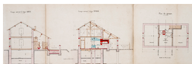
Dérivation de Conflandey : maison éclusière (1876). Phot. Jérôme Mongreville, Autr. Charles Marie Albert Travelet IVR43_20207000164NUC4A
