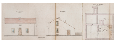
Dérivation de Conflandey : maison éclusière (1876). Phot. Jérôme Mongreville, Autr. Charles Marie Albert Travelet IVR43_20207000162NUC4A
