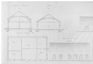
Jean Schmitt, industriel à Thann. Demande en autorisation d'établir une usine de teinture, blanchiment et impression sur écheveaux [plan, coupe et élévation des dépendances et bureaux]. Phot. Jérôme Mongreville, Phot. Eugène Bédaton IVR43_20019000241X
