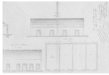
Jean Schmitt, industriel à Thann. Demande en autorisation d'établir une usine de teinture, blanchiment et impression sur écheveaux [plan et élévation des séchoirs]. Phot. Jérôme Mongreville, Phot. Eugène Bédaton IVR43_20019000237X
