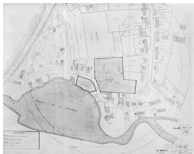
Etablissement J. Beauseigneur à Danjoutin (Territoire de Belfort) Ancienne Teinturerie Alsacienne - Plan d'ensemble de la propriété. Phot. Jérôme Mongreville, Phot. Théophile Moritz IVR43_20019000007V
