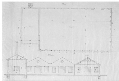
Jean Schmitt, industriel à Thann. Demande en autorisation d'établir une usine de teinture, blanchiment et impression sur écheveaux [plan et élévation de la teinturerie]. Phot. Jérôme Mongreville, Phot. Eugène Bédaton IVR43_20019000236X
