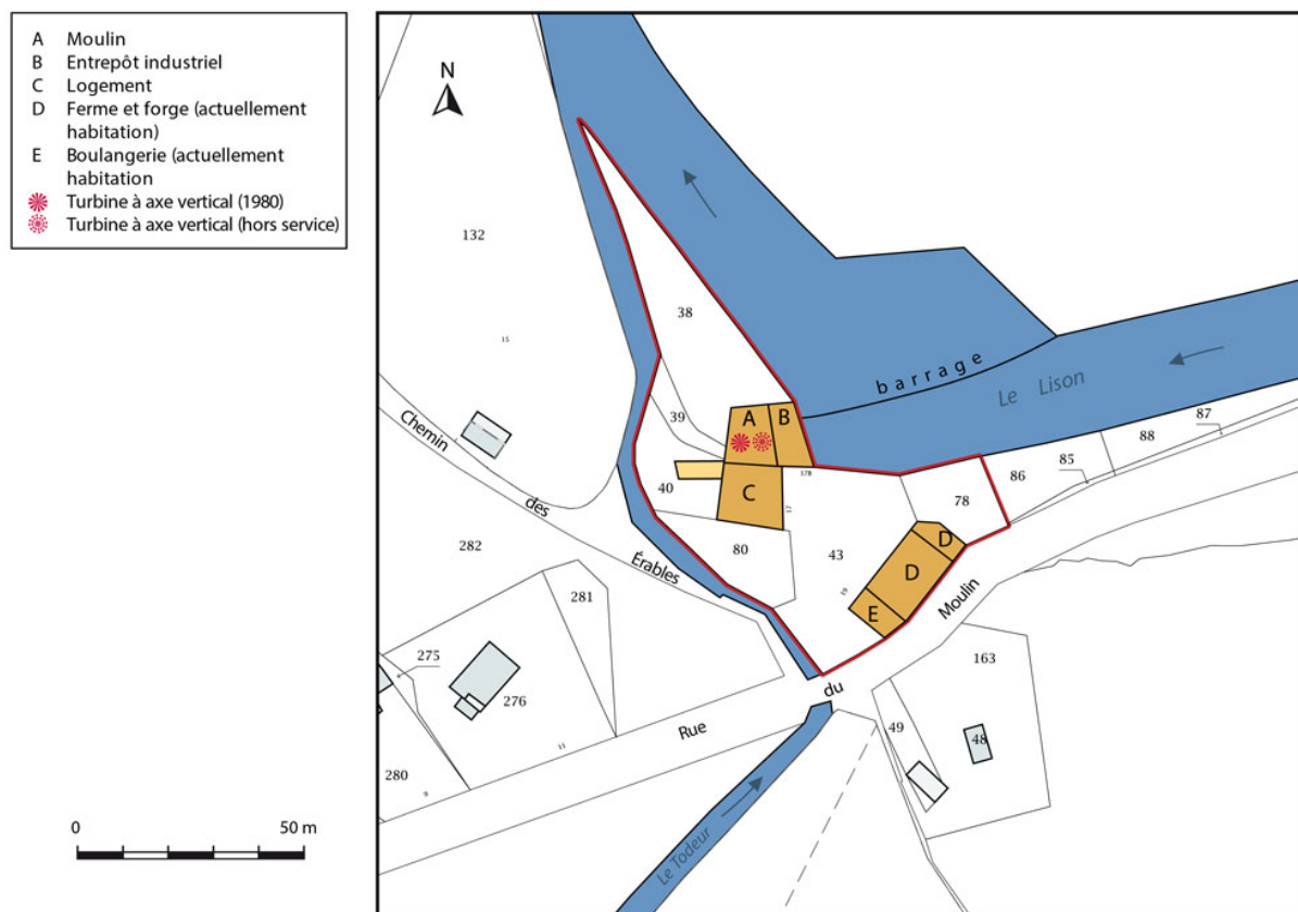
Plan-masse et de situation. Extrait du plan cadastral, 2016, section ZB.
