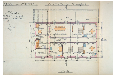
Société coopérative de fromagerie de Frasne. Construction d'une fromagerie, étage, 1926. Phot. Jérôme Mongreville IVR43_20182500158NUC4A
