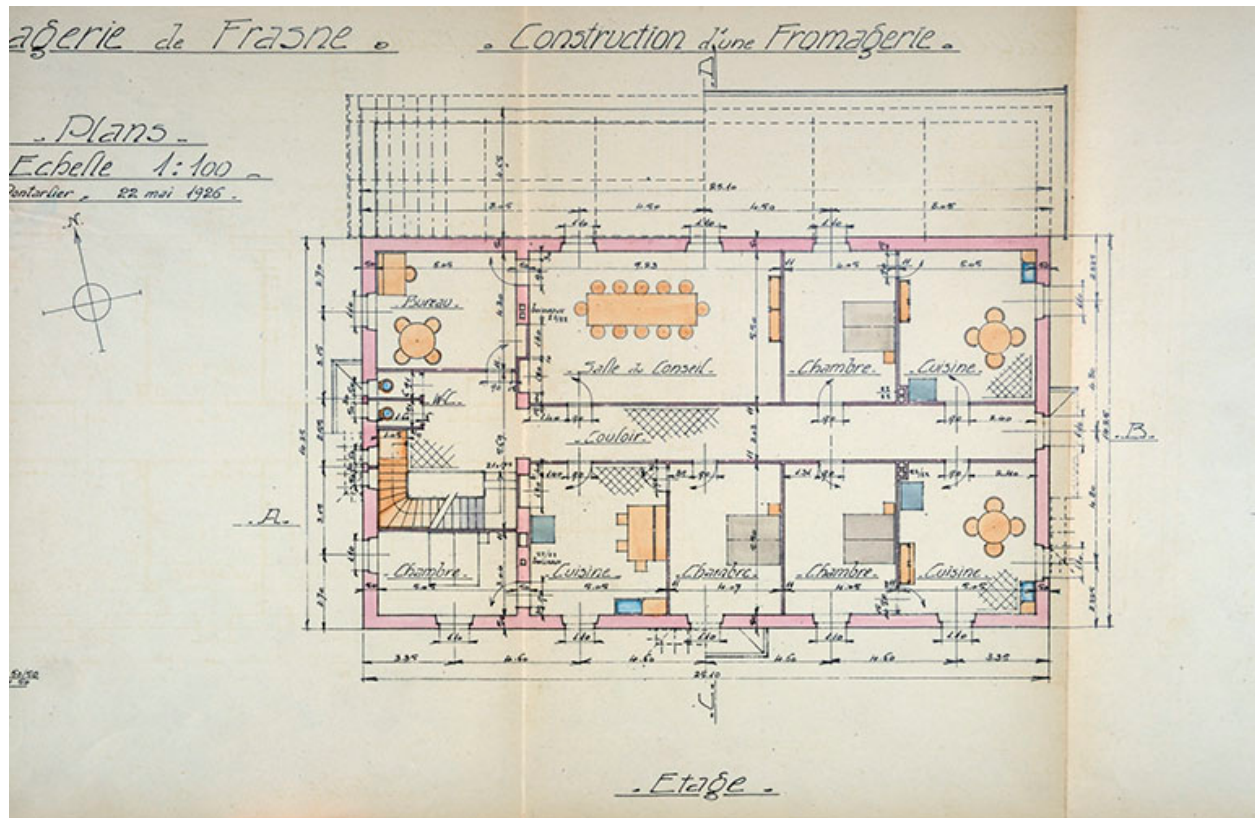
Société coopérative de fromagerie de Frasne. Construction d'une fromagerie, étage, 1926.
