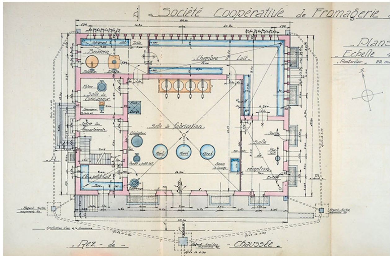
Société coopérative de fromagerie de Frasne. Construction d'une fromagerie, rez-de-chaussée, 1926.
