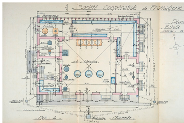
Société coopérative de fromagerie de Frasne. Construction d'une fromagerie, rez-de-chaussée, 1926. Phot. Jérôme Mongreville IVR43_20182500157NUC4A
