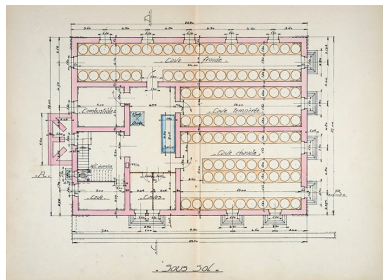
Société coopérative de fromagerie de Frasne. Construction d'une fromagerie, sous-sol, 1926. Phot. Jérôme Mongreville IVR43_20182500156NUC4A
