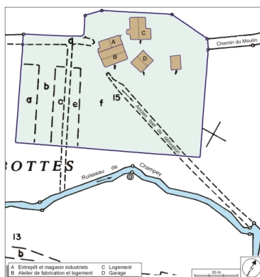
Plan-masse et de situation. Extrait du plan cadastral numérisé, 2005, section ZA, 1:2000 agrandi à 1:1000. Dess. André Céréza IVR43_20067000038NUDA
