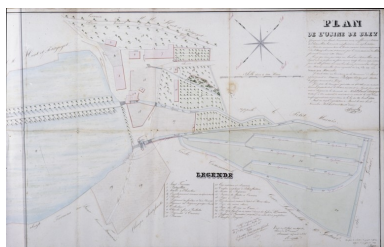
Plan de l'usine de Bley composée d'un haut fourneau avec souffleries à pistons, de patouillets [...]. Phot. Yves Sancey, Autr. Gonzalez IVR43_19877000018XA
