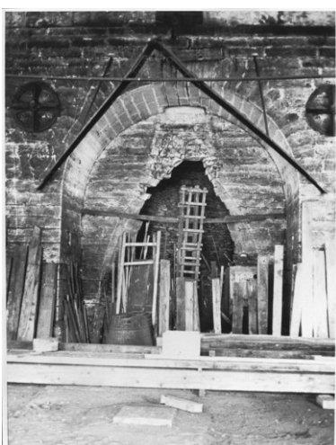
Détail de la base de la tour du haut fourneau vers 1960. Phot. Yves Sancey IVR43_19897000882X
