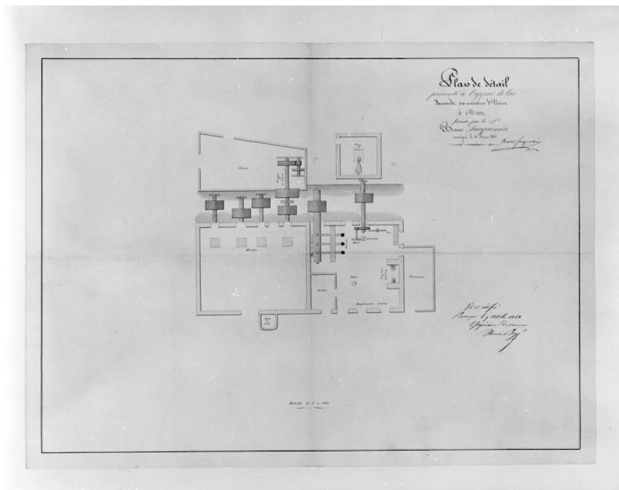
Plan de détail présenté à l'appui de la demande en maintien d'usine à Morez formée par le Sr Bruno Jacquemin. Dessin, 1841. Echelle 1:100.
