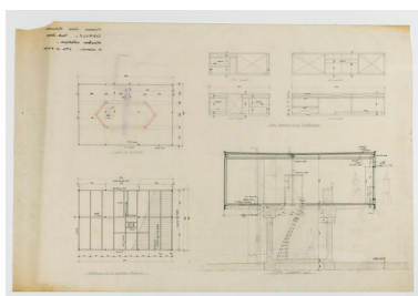
Schémas et plans de la villa. Phot. Sonia Dourlot IVR43_20167001432NUC4A
