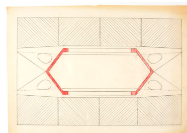
Dessin du coffrage de la base (pile) montrant la sous-face du premier étage, André Maisonnier, s.d. Phot. Sonia Dourlot IVR43_20177000550NUC2A
