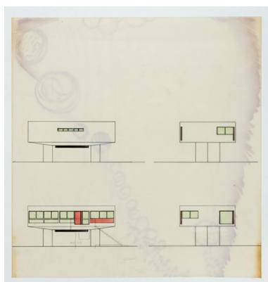
Plans en élévation des quatre faces de la maison. Phot. Sonia Dourlot IVR43_20167001431NUC4A
