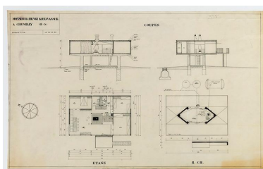
Plans en coupe de la villa. Phot. Sonia Dourlot IVR43_20167001429NUC4A
