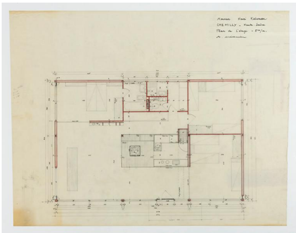
Plan en coupe de l'étage.
