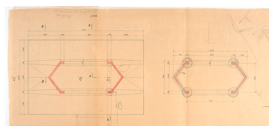
Cahier de coffrage et armature de la structure de la pile, André Maisonnier, s.d. Phot. Sonia Dourlot IVR43_20177000555NUC2A
