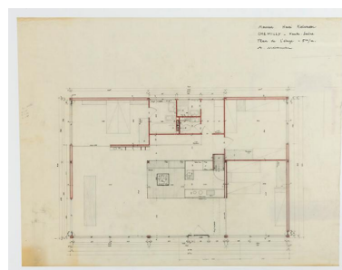
Plan en coupe de l'étage. Phot. Sonia Dourlot IVR43_20167001433NUC4A
