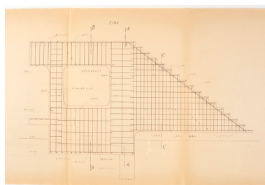
Cahier de coffrage et armature de la structure de l'escalier, s.d. Phot. Sonia Dourlot IVR43_20177000553NUC2A
