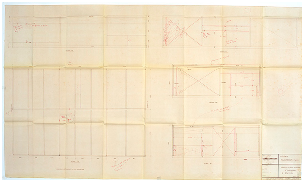
Plan de la charpente métallique avec annotations de l'entreprise Waltefaugle, André Maisonnier, 1er septembre 1966.
