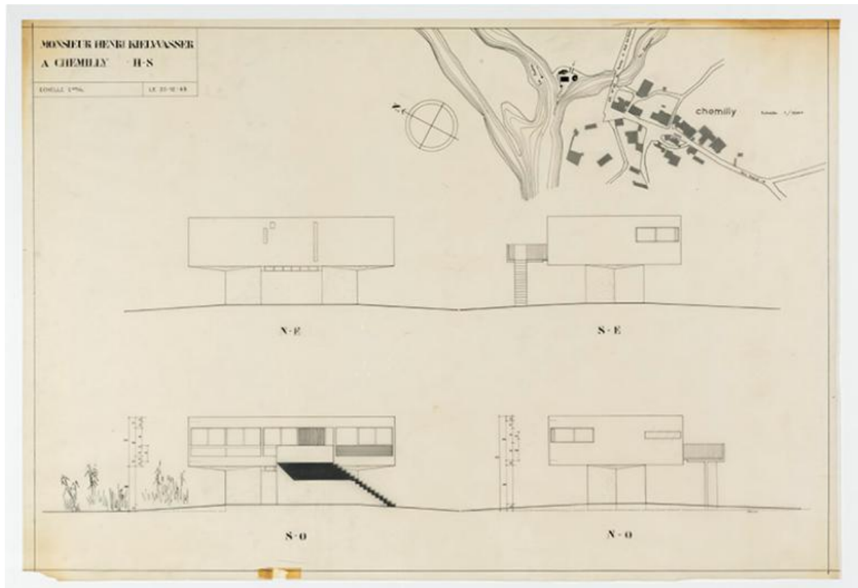
Plans en élévation des quatre faces de la maison et extrait de plan cadastral.
