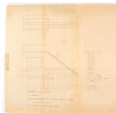
Cahier de coffrage et armature de la structure de l'escalier, s.d. Phot. Sonia Dourlot IVR43_20177000552NUC2A
