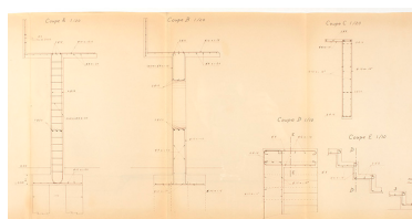
Cahier de coffrage et armature de la structure de l'escalier, André Maisonnier, s.d. Phot. Sonia Dourlot IVR43_20177000554NUC2A
