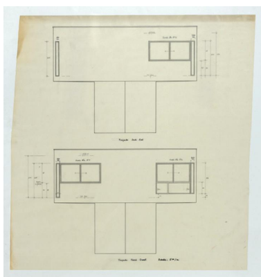
Plans en élévation des faces Nord et Sud. Phot. Sonia Dourlot IVR43_20167001438NUC4A
