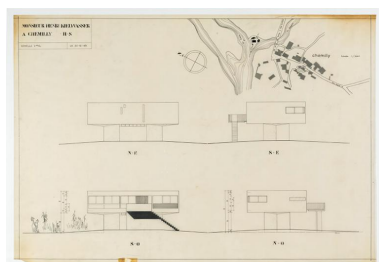
Plans en élévation des quatre faces de la maison et extrait de plan cadastral. Phot. Sonia Dourlot IVR43_20167001428NUC4A
