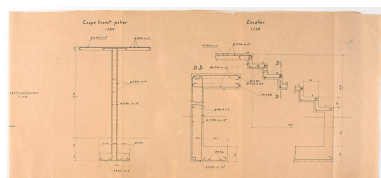
Cahier de coffrage et armature de la structure de l'escalier, s.d. Phot. Sonia Dourlot IVR43_20177000560NUC2A
