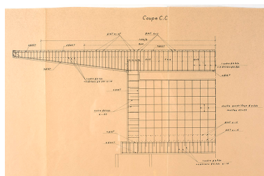
Cahier de coffrage et armature de la structure : ferailage de la dalle, André Maisonnier, s.d.
