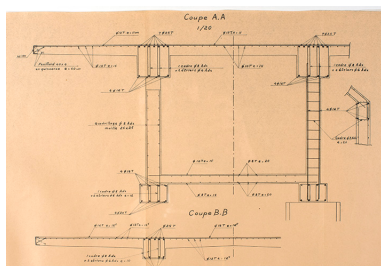
Cahier de coffrage et armature de la structure de l'escalier, s.d. Phot. Sonia Dourlot IVR43_20177000552NUC2A
