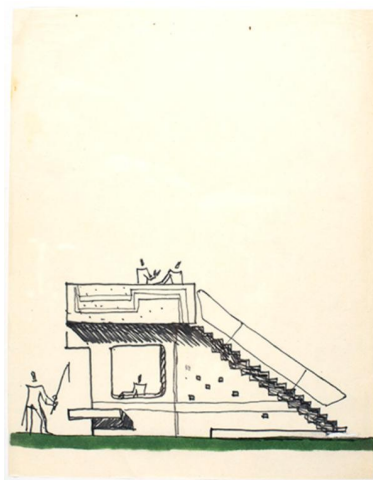
Esquisse en élévation de l'escalier extérieur, André Maisonnier, s.d., ca. 1960-1965, Archives privées. Phot. Sonia Dourlot IVR43_20177000549NUC2A
