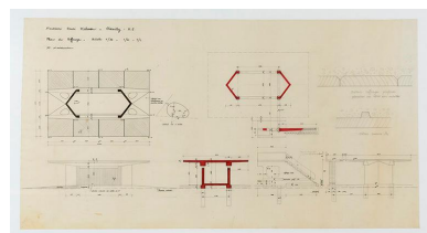
Plan en coupe du coffrage de la pile de la maison Phot. Sonia Dourlot IVR43_20167001430NUC4A
