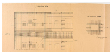
Cahier de coffrage et armature de la structure : ferailage de la dalle, André Maisonnier, s.d.
