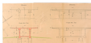
Cahier de coffrage et armature de la structure de la pile et du plancher du premier étage, s.d. Phot. Sonia Dourlot IVR43_20177000556NUC2A
