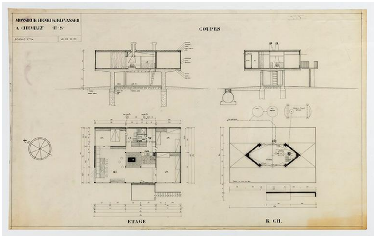
Plans en coupe de la villa.
