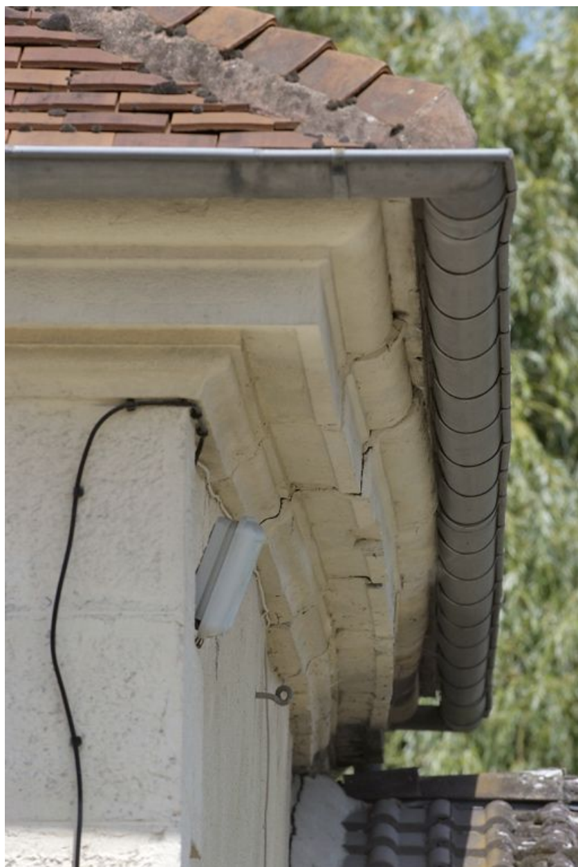
Détail de maçonnerie : la corniche en pierre de taille.
