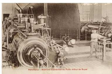
Ronchamp. - Machine d'Extraction du Puits Arthur de Buyer. Phot. Jérôme Mongreville IVR43_20057000633NUCA
