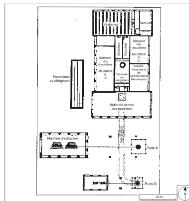
Plan-masse au début du 20e siècle. Dess. André Céréza IVR43_20087000282NUDA
