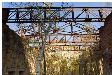
Bâtiment des bureaux et de la lampisterie : éléments de la charpente métallique. Phot. Jérôme Mongreville IVR43_20077000591NUCA
