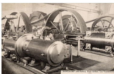
Ronchamp (Hte-Saône). - Puits Arthur. Les ventilateurs. Phot. Jérôme Mongreville IVR43_20057000634NUCA
